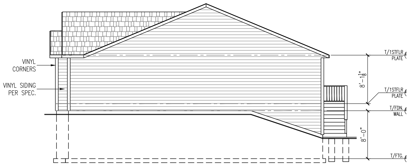
ELEVATION 1 RIGHT ELEVATION SCALE: 1/8" = 1'-0"
