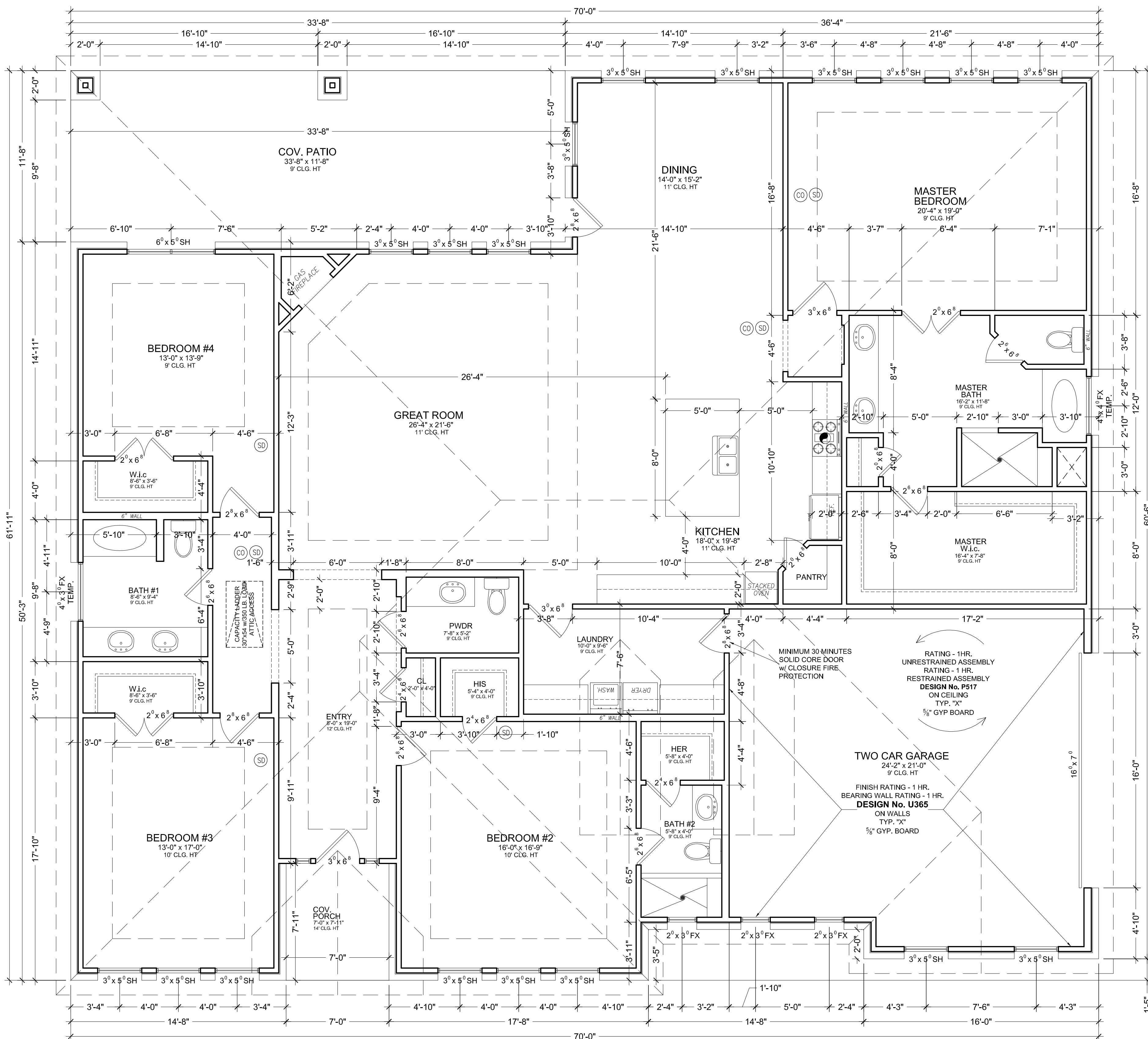
SCALE: 1/4" = 1'-0"
