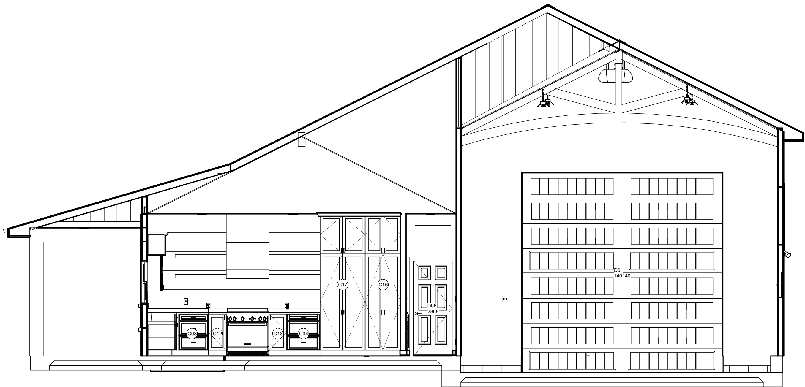
Elevation 12
