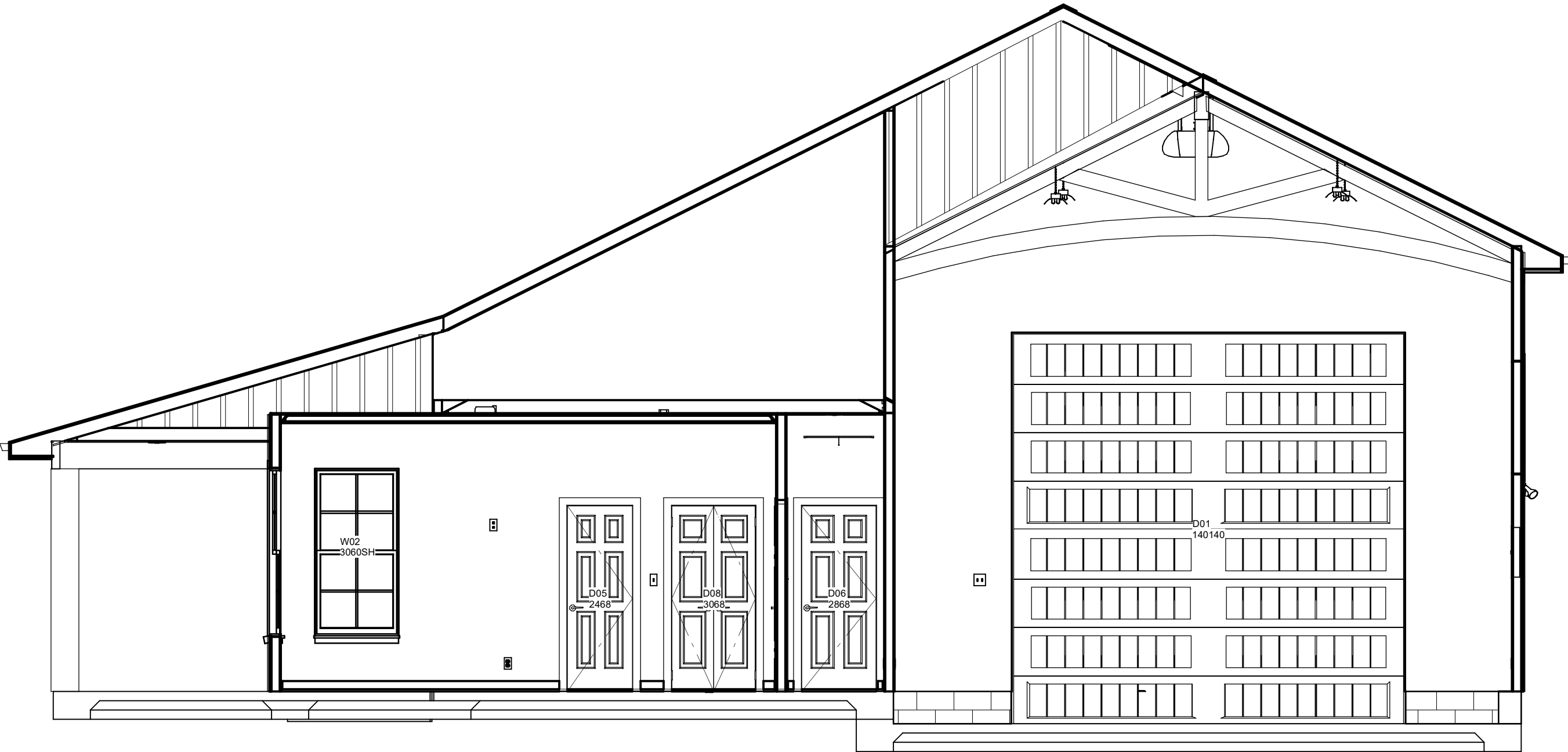
Elevation 5
